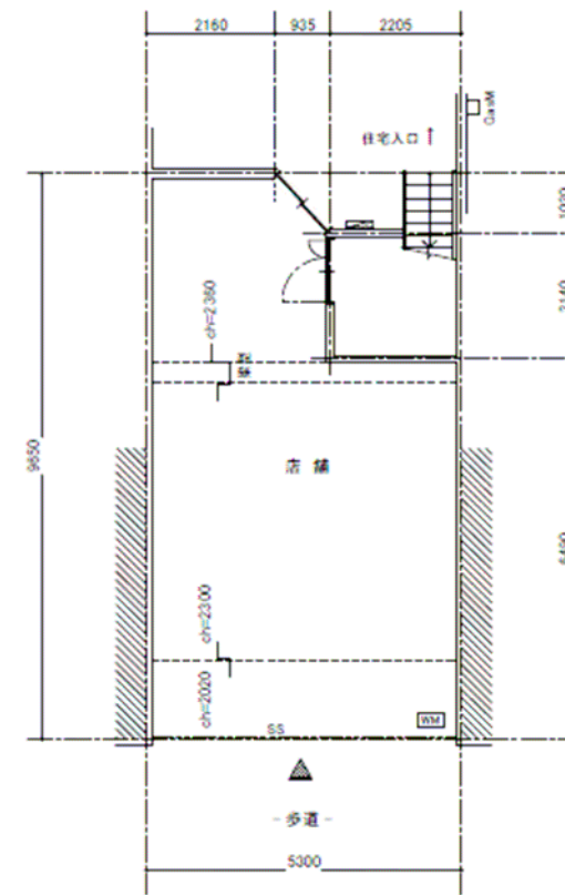
店舗部分のみ作図
