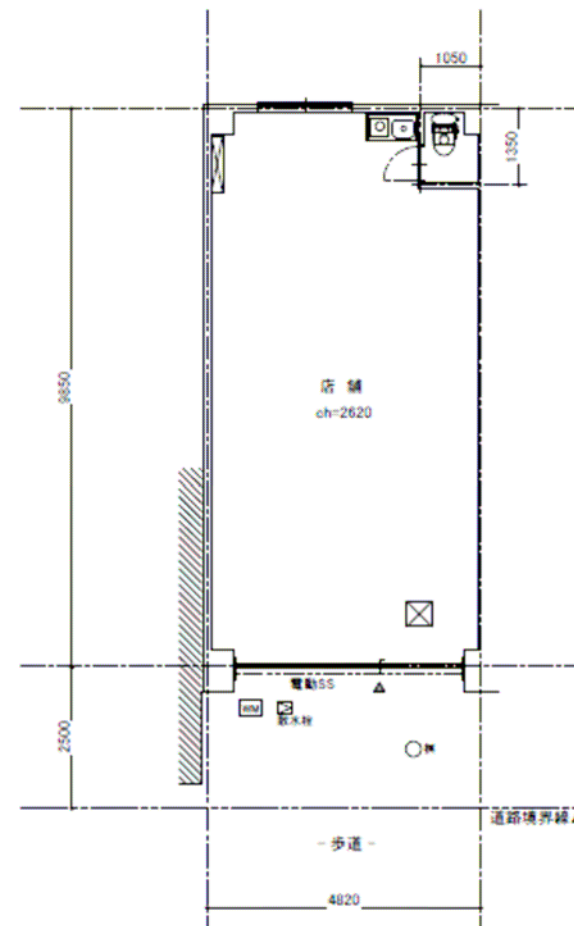
- 1F 平面図 -
