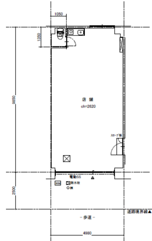
- 1F 平面図 -
